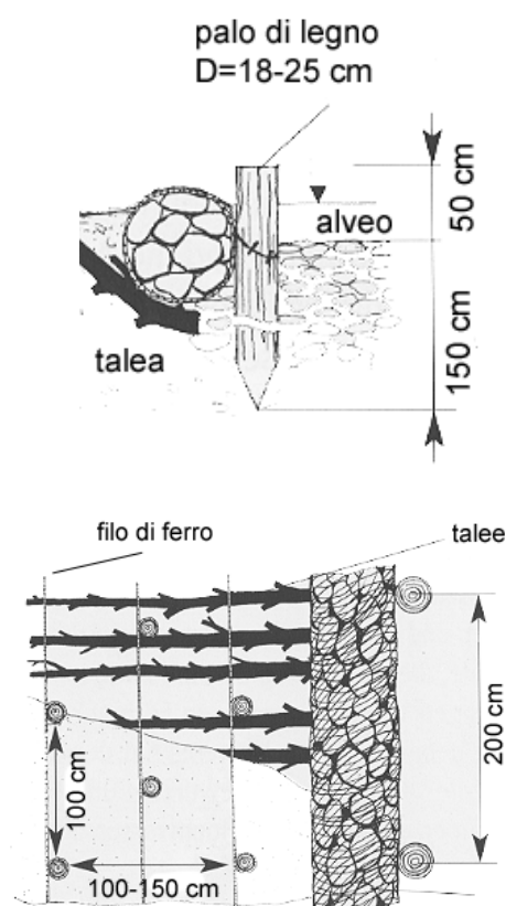
Figura 2.4 - Copertura diffusa (da Provincia di Terni, 2003-mod.); Dettaglio del presidio al piede (da Florineth, 2004-mod.)
