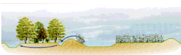
Figura 2.25 - Esempio di risezionamento dell'alveo con creazione di golenale vegetata su una sponda
