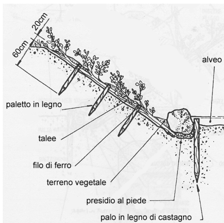
Figura 2.4 - Copertura diffusa (da Provincia di Terni, 2003-mod.); Dettaglio del presidio al piede (da Florineth, 2004-mod.)
