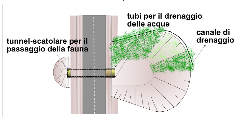
Figura 2.32 - Esempio di realizzazione di sottopasso in cui è necessario il risezionamento del versante in sezione a) e b) e visto dall'alto con indicazione di recupero a verde di metà versante (speculare) c)
