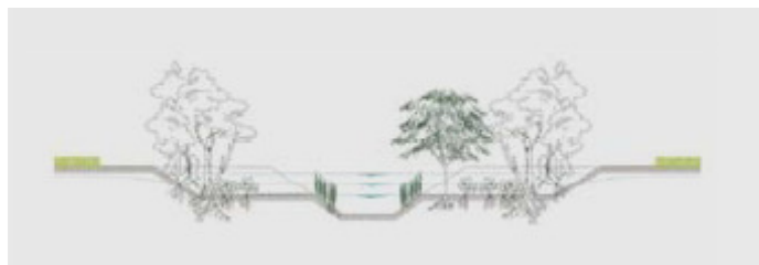
Fig. 3-7 - Risezionamento di alveo con inserimento di vegetazione su entrambe le sponde
