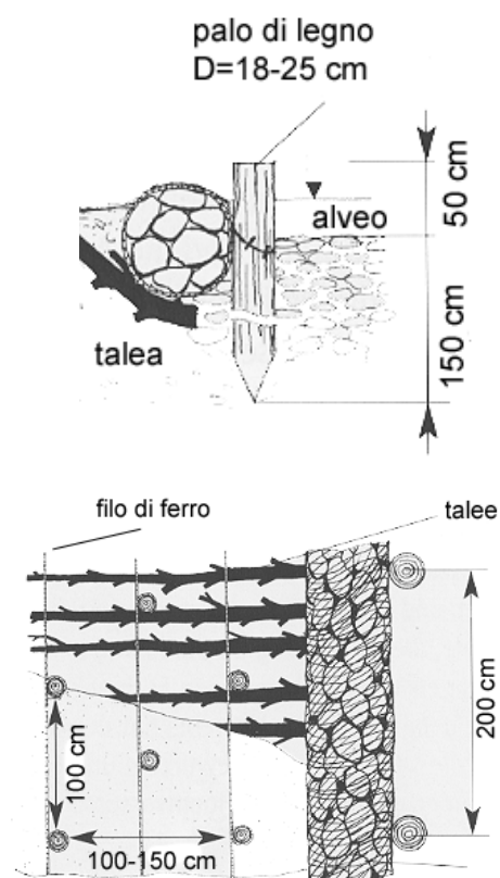
Fig. 3-1 - Copertura diffusa (da Provincia di Terni, 2003-mod.); Dettaglio del presidio al piede (da Florineth, 2004-mod.)
