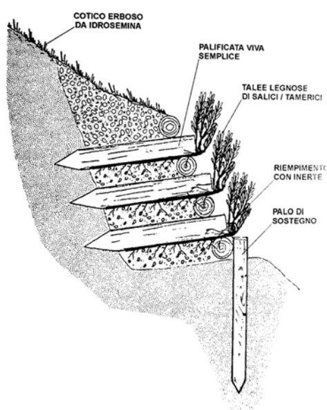
Palificata in legname con talee a parete semplice
