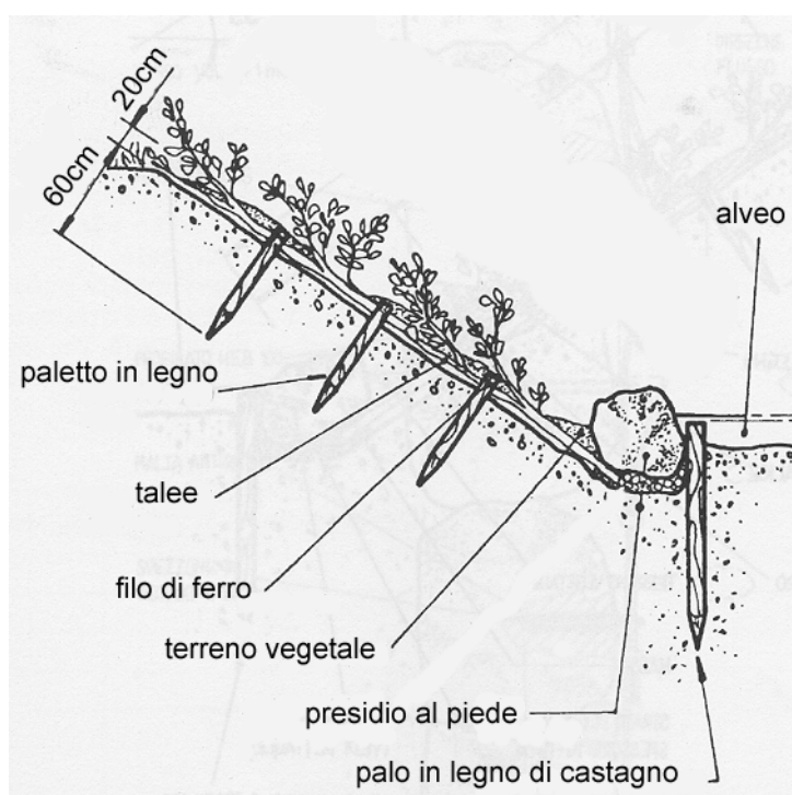
Fig. 3-1 - Copertura diffusa (da Provincia di Terni, 2003-mod.); Dettaglio del presidio al piede (da Florineth, 2004-mod.)
