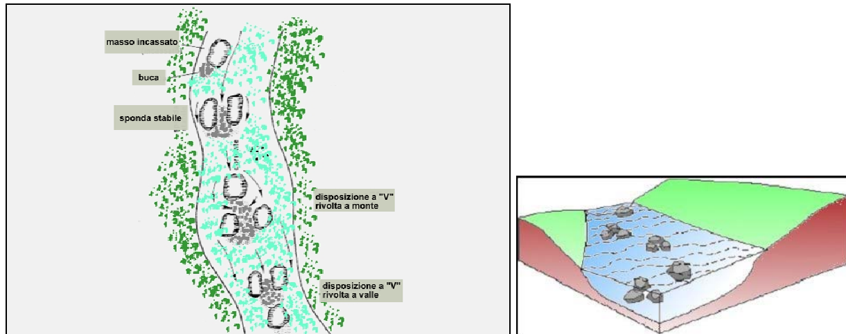
Figura 2.21 - Esempio di sistemazione di massi in alveo al fine di garantire una maggior disponibilità di habitat per gli organismi acquatici e una maggiore ritenzione del detrito
